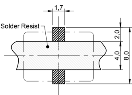
Scale - 3:1
